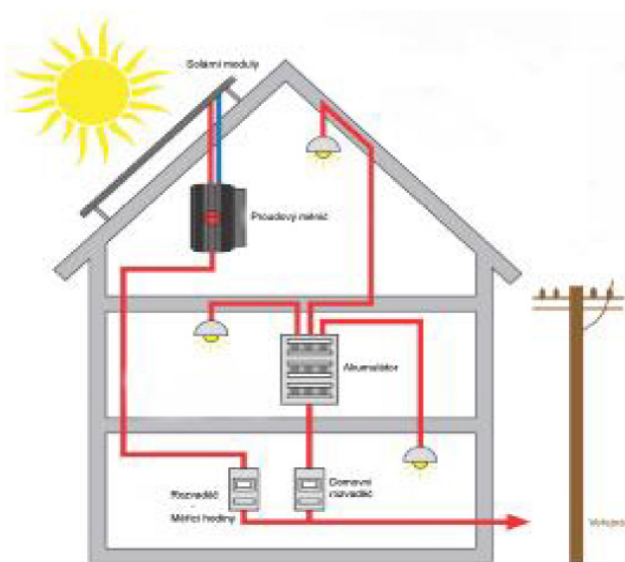
Obr.1.: Princip zapojení fotovoltaického zdroje u rodinného domu
